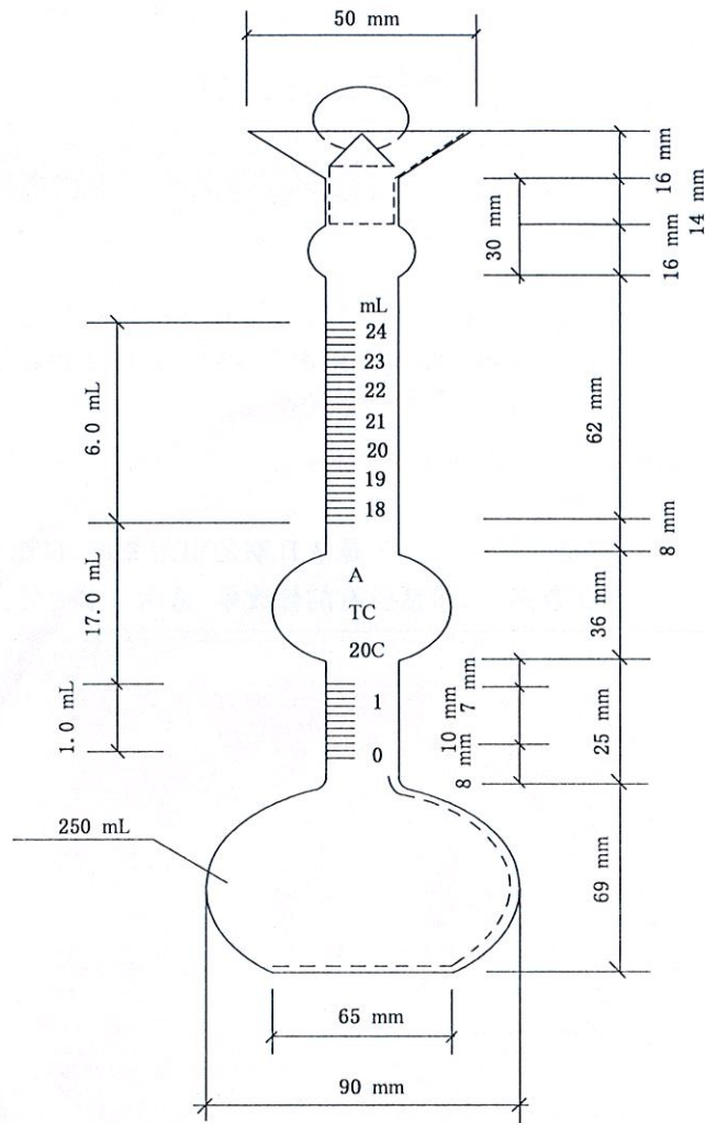
图 1 李氏瓶示意图
